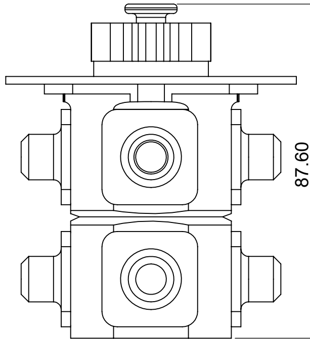
ANDAIR FS2020-D2 MASS 353g
